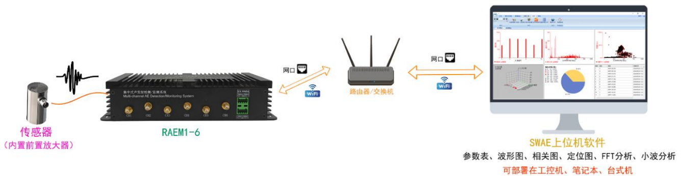
内置前置放大器的传感器连接
